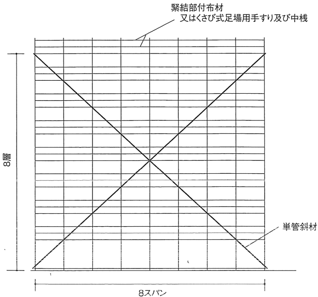
図-30 単管による取付け例
