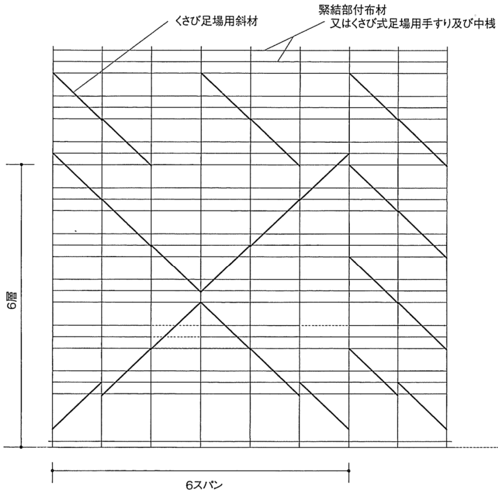
図-31 専用斜材による取付け例
