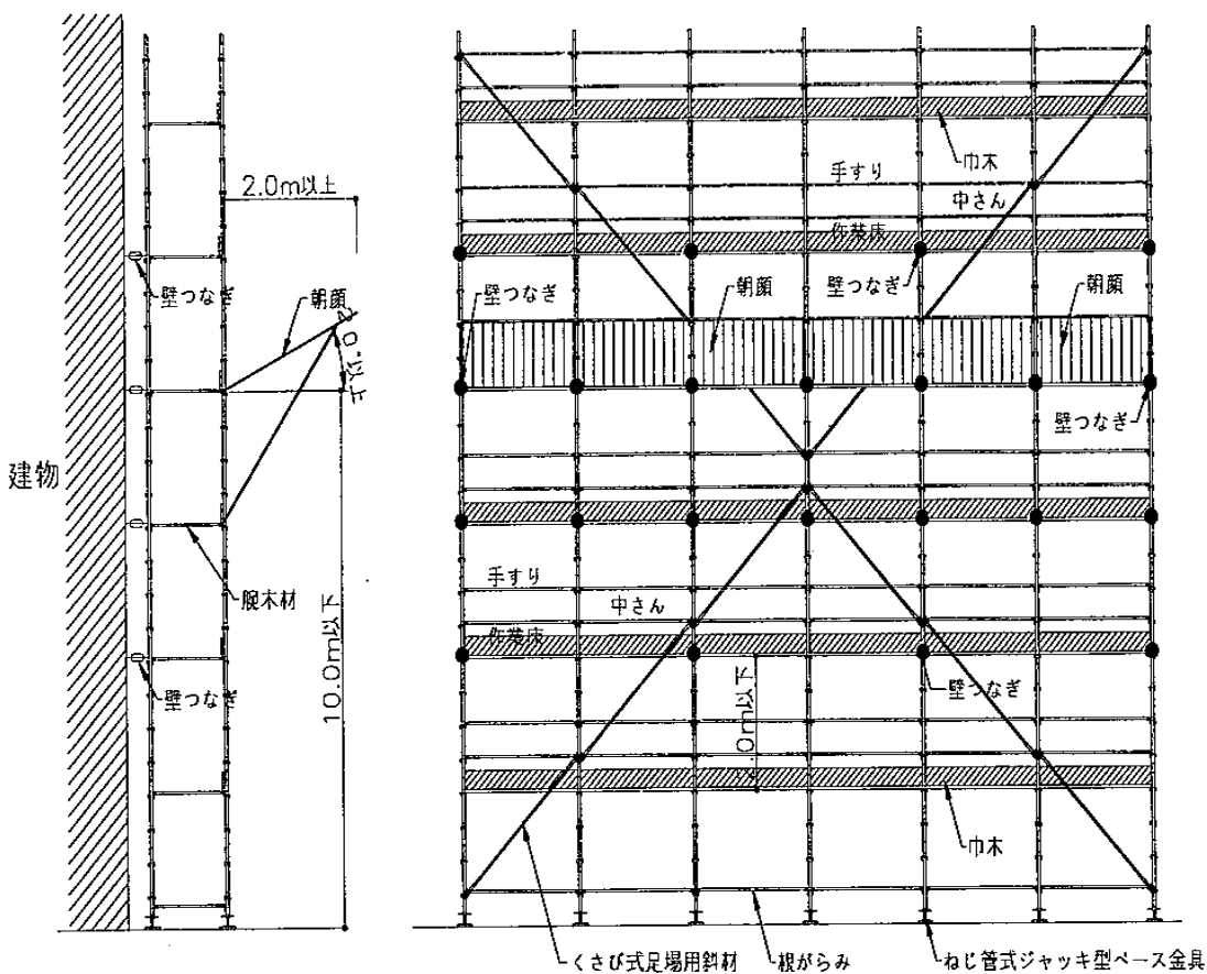
朝顔の取付例
